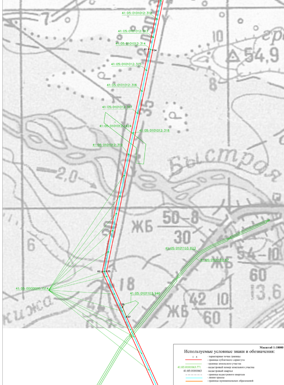
Графическое описание местоположения границ публичного сервитута в отношении земель и земельных участков для их использования в целях эксплуатации (размещения) линейного объекта: Сооружение ВЛЭП 110кВ на металлических опорах (Елизово II - Авача II - Сосновка II - Советская II), кадастровый номер объекта 41:05:0000000:823
