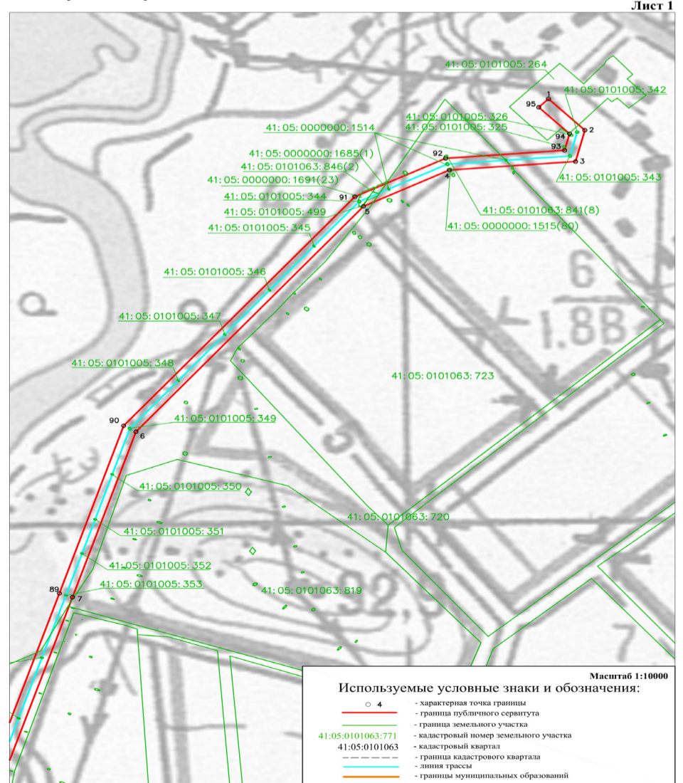
Графическое описание местоположения границ публичного сервитута в отношении земель и земельных участков для их использования в целях эксплуатации (размещения) линейного объекта: Сооружение ВЛЭП 110кВ на металлических опорах (Елизово II - Авача II - Сосновка II - Советская II), кадастровый номер объекта 41:05:0000000:823
