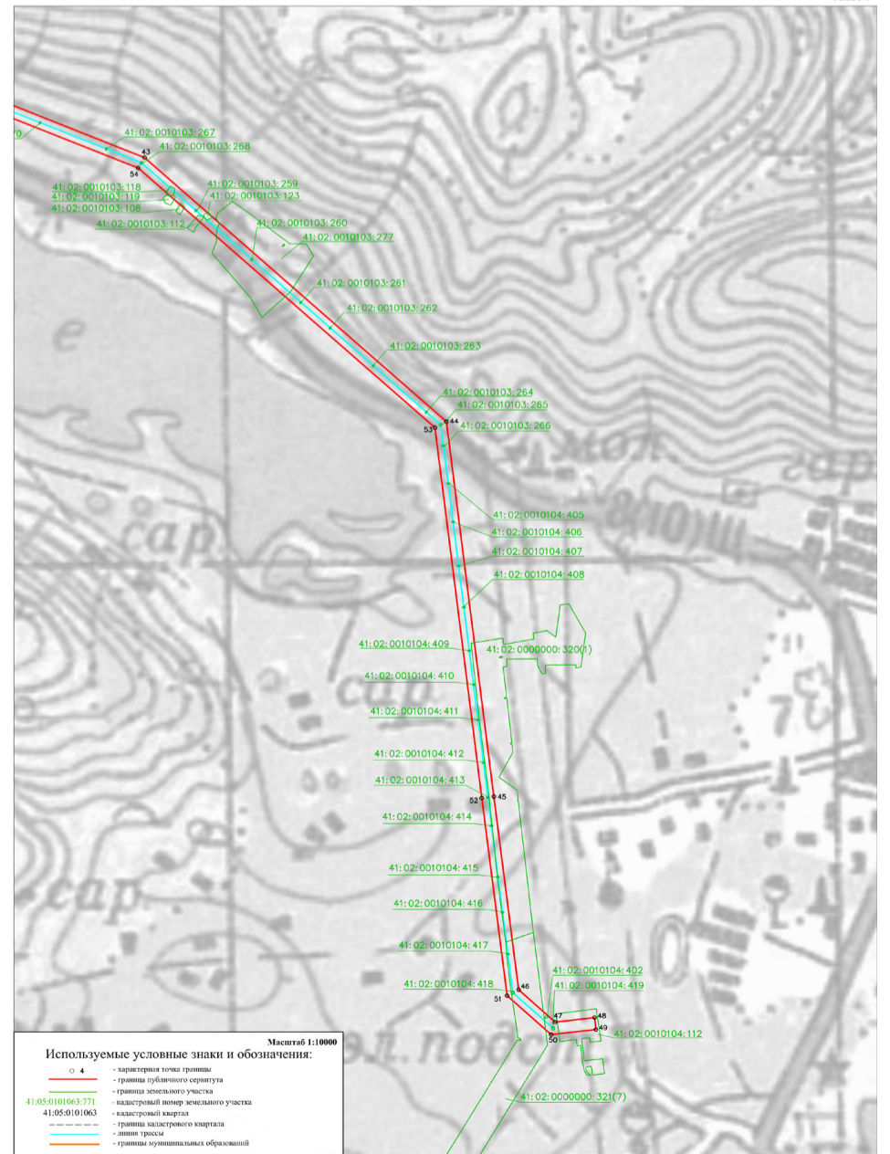
Графическое описание местоположения границ публичного сервитута в отношении земель и земельных участков для их использования в целях эксплуатации (размещения) линейного объекта: Сооружение ВЛЭП 110кВ на металлических опорах (Елизово II - Авача II - Сосновка II - Советская II), кадастровый номер объекта 41:05:0000000:823
