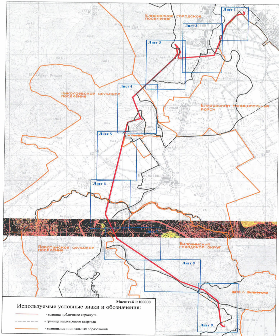
Графическое описание местоположения границ публичного сервитута в отношении земель и земельных участков для их использования в целях эксплуатации (размещения) линейного объекта: Сооружение ВЛЭП 110кВ на металлических опорах (Елизово II - Авача II - Сосновка II - Советская II) кадастровый номер объекта 41:05:0000000:823
